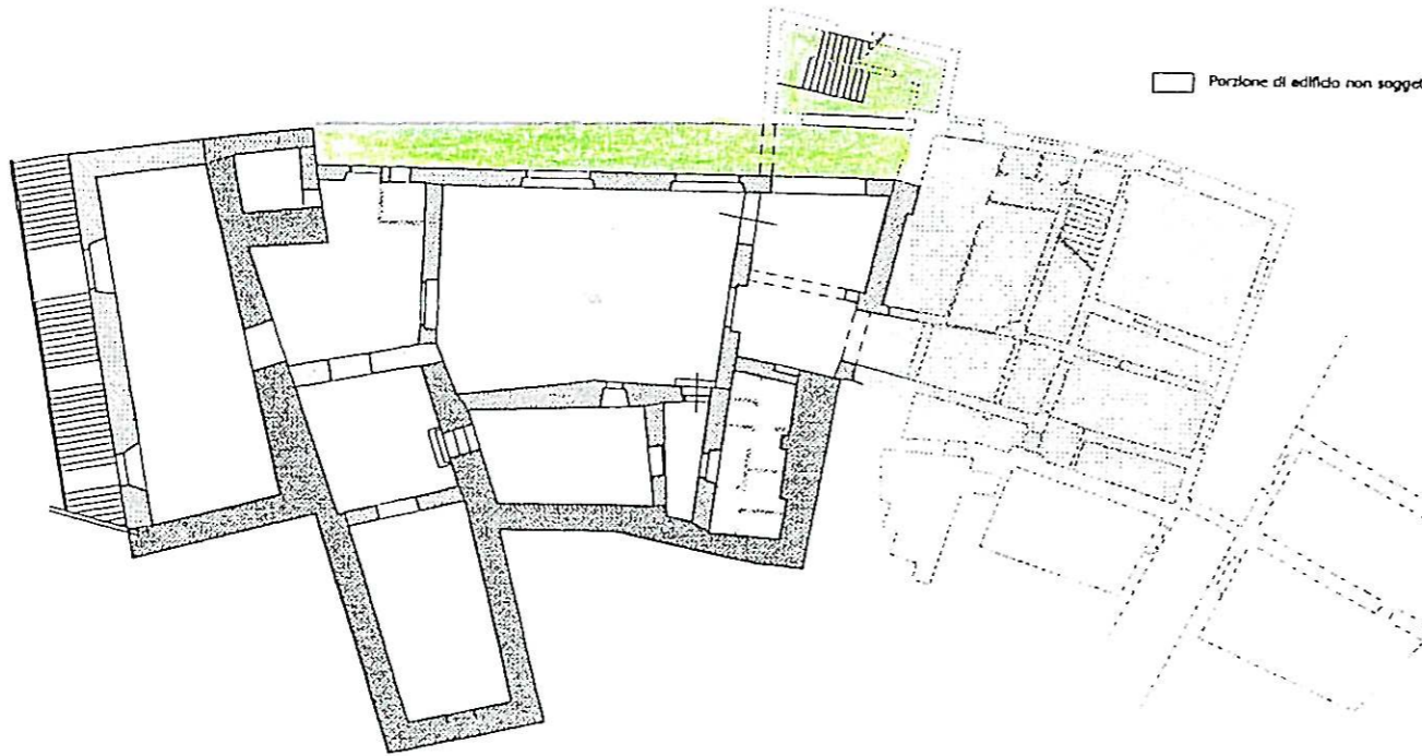
PLANIMETRIA PIANO INTERRATO
