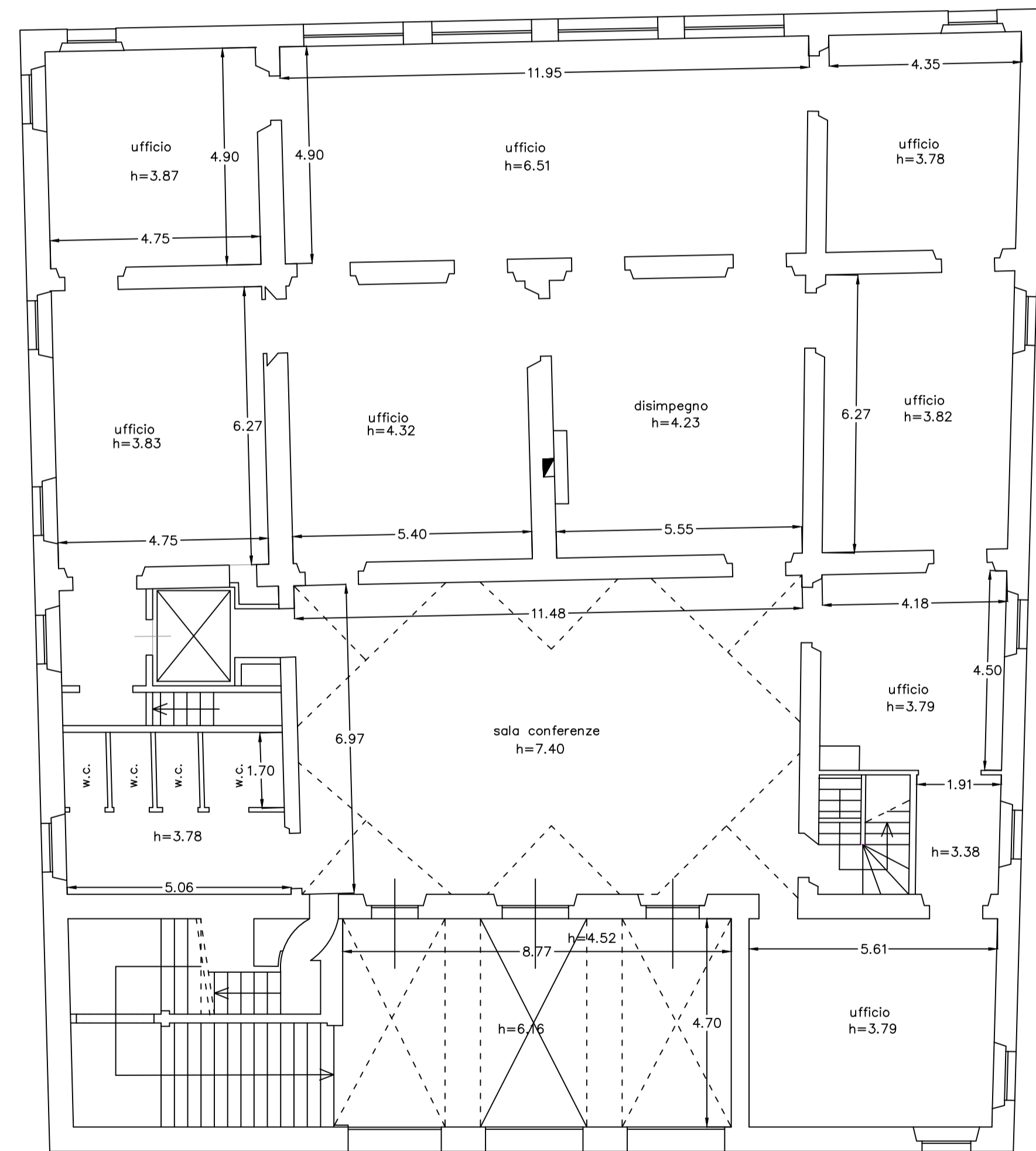
PIANO PRIMO scala 1:100
