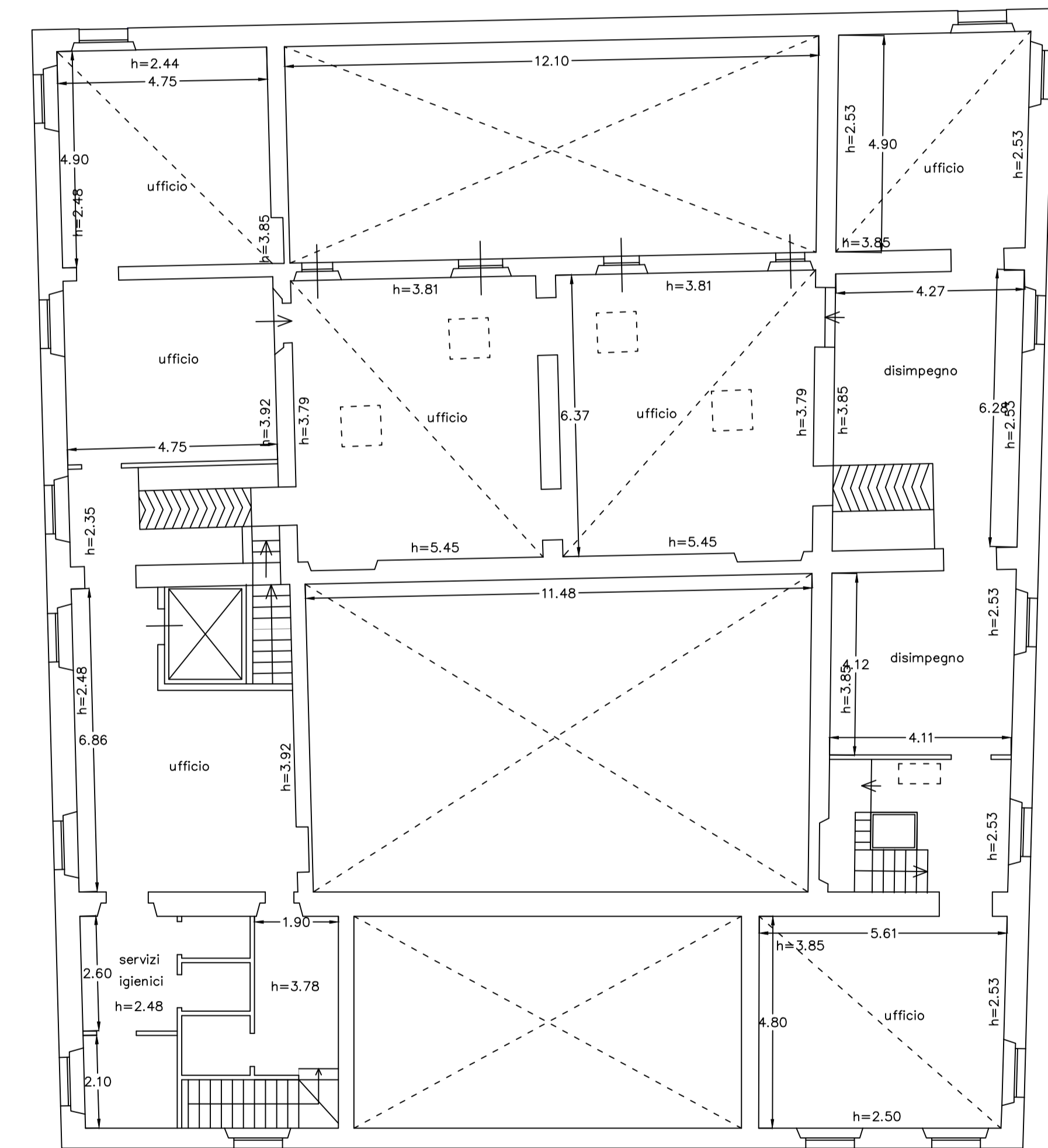
PIANO SECONDO scala 1:100
