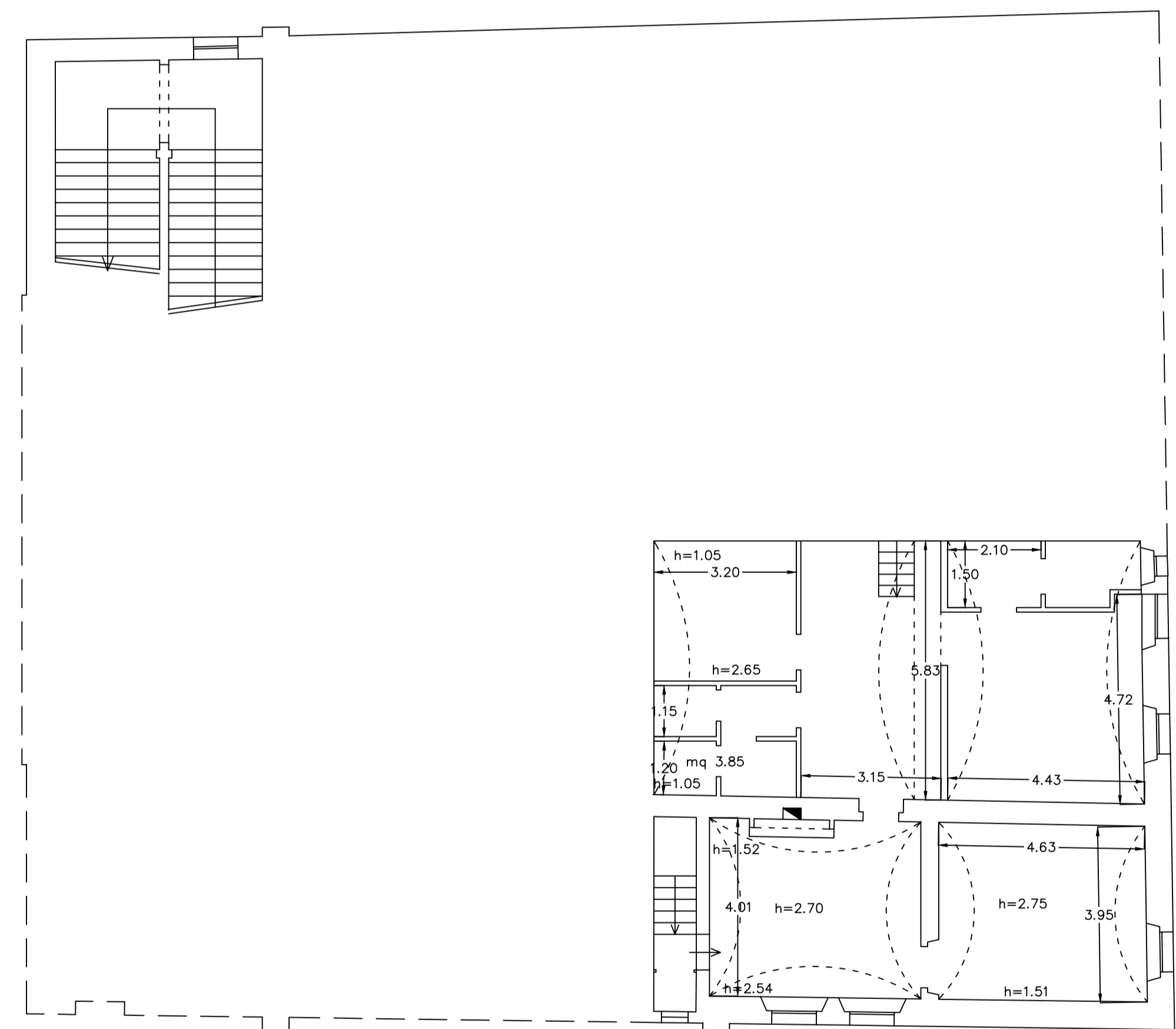
PIANO RIALZATO scala 1:100
