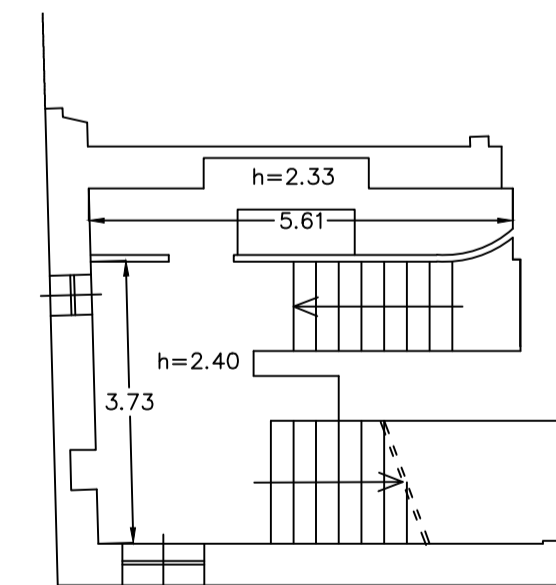
PIANO PRIMO MEZZANINO scala 1:100
