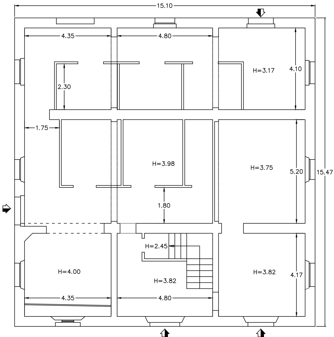
FABBRICATO PRINCIPALE PIANO TERRA scala 1:100
