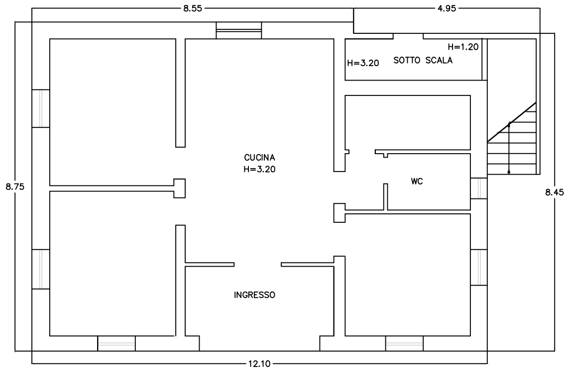
EDIFICIO PRINCIPALE PIANO TERRA Scala 1:100
