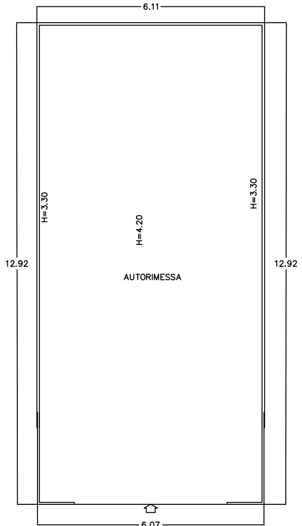
AUTORIMESSA SUB. 3 Scala 1:100
