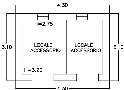
ANNESSE SUB. 1 Scala 1:100
