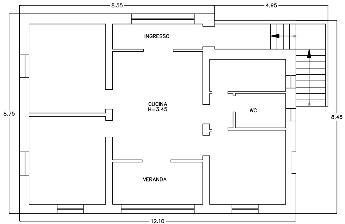
EDIFICIO PRINCIPALE PIANO PRIMO Scala 1:100
